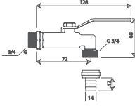
3/4 Kollu Küresel Bahçe Musluğu
