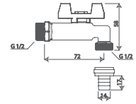
1/2 Kelebek Küresel Bahçe Musluğu
